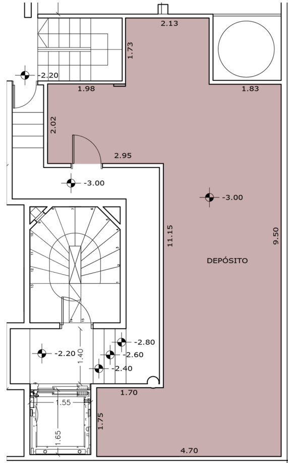
Subsuelo
